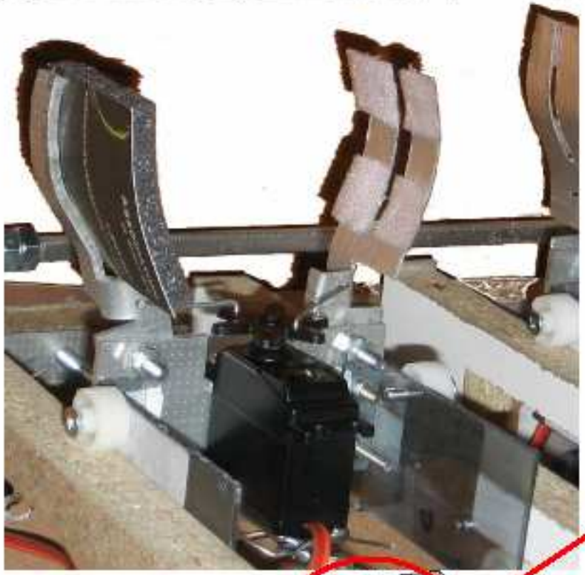
Pince avant : manipulation des palets.
